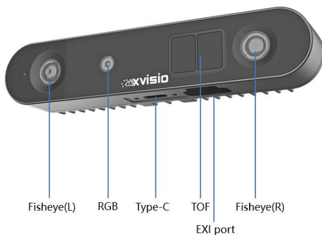
图 1-1 SeerSense™ DS80 系列产品示意
