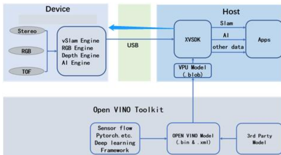
图 3-9 AI(CNN)引擎整体架构
