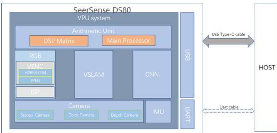
图 2-1 内部单元框图
